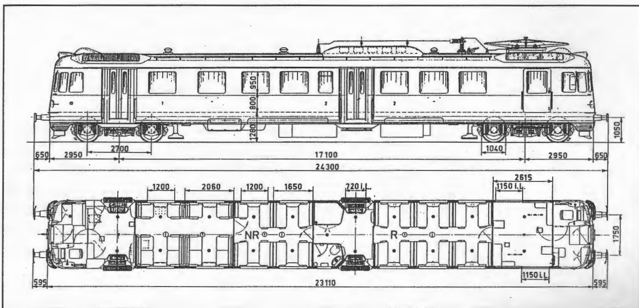
ABDe 4/4 11 bis 15
